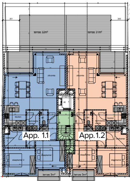
VERDIEPING 1
