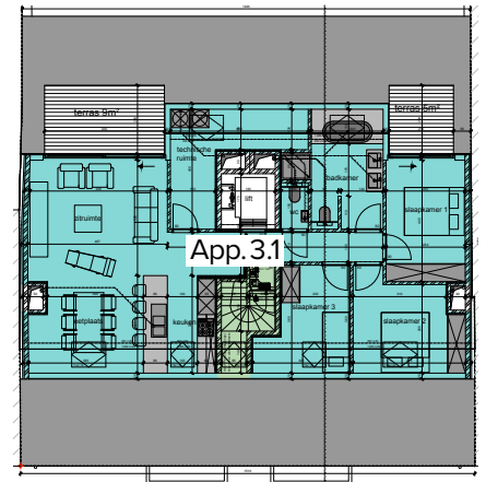
VERDIEPING 3
