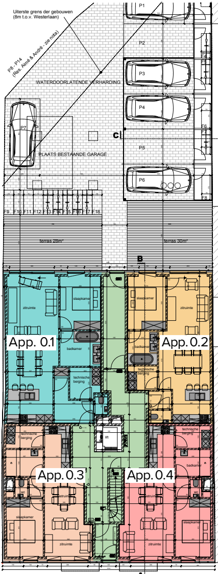
GELIJKVLOERS
